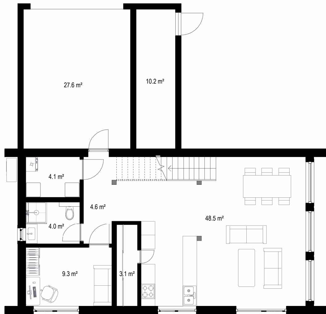
1.STĀVA PLĀNS
