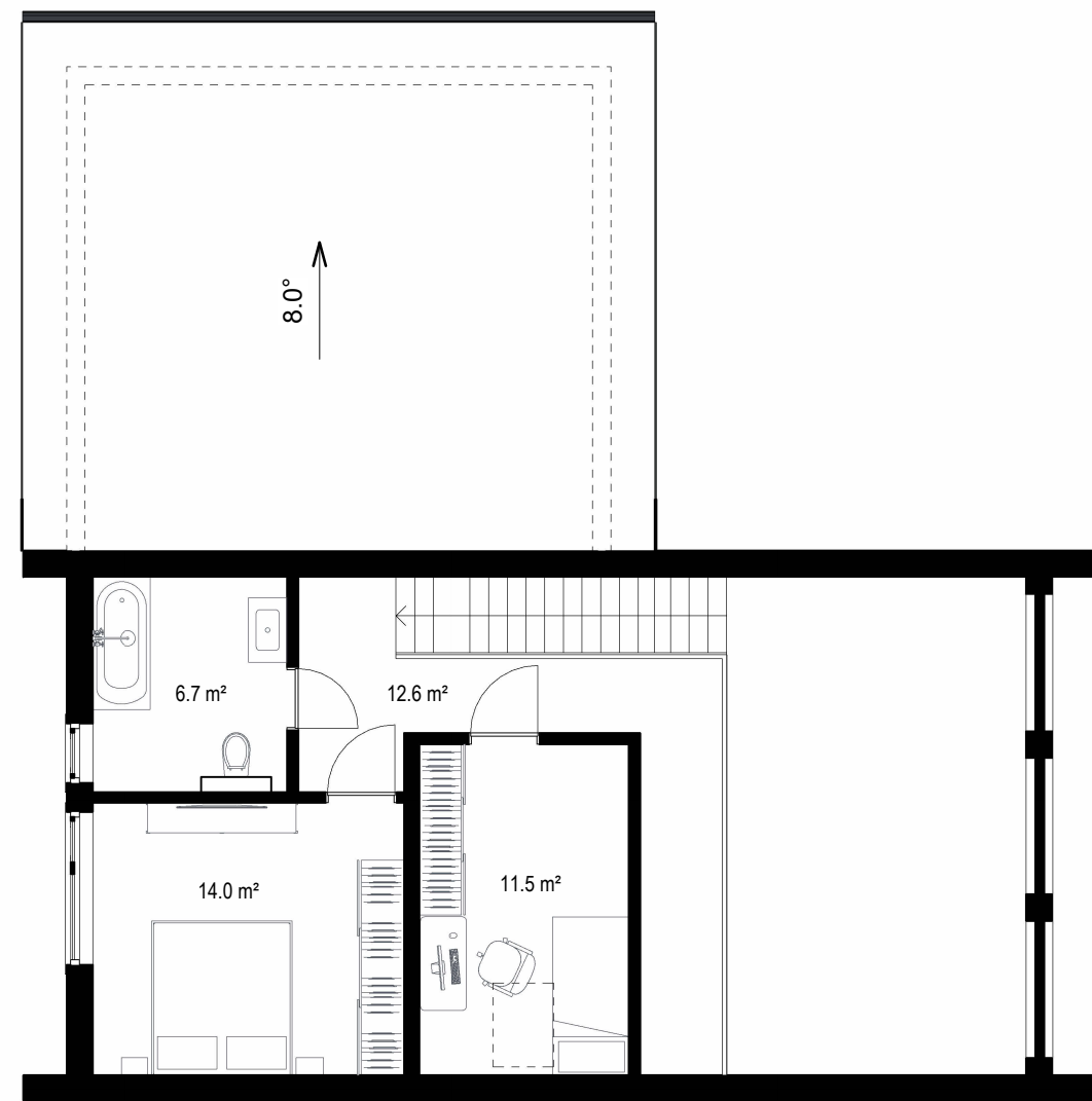
2.STĀVA PLĀNS
